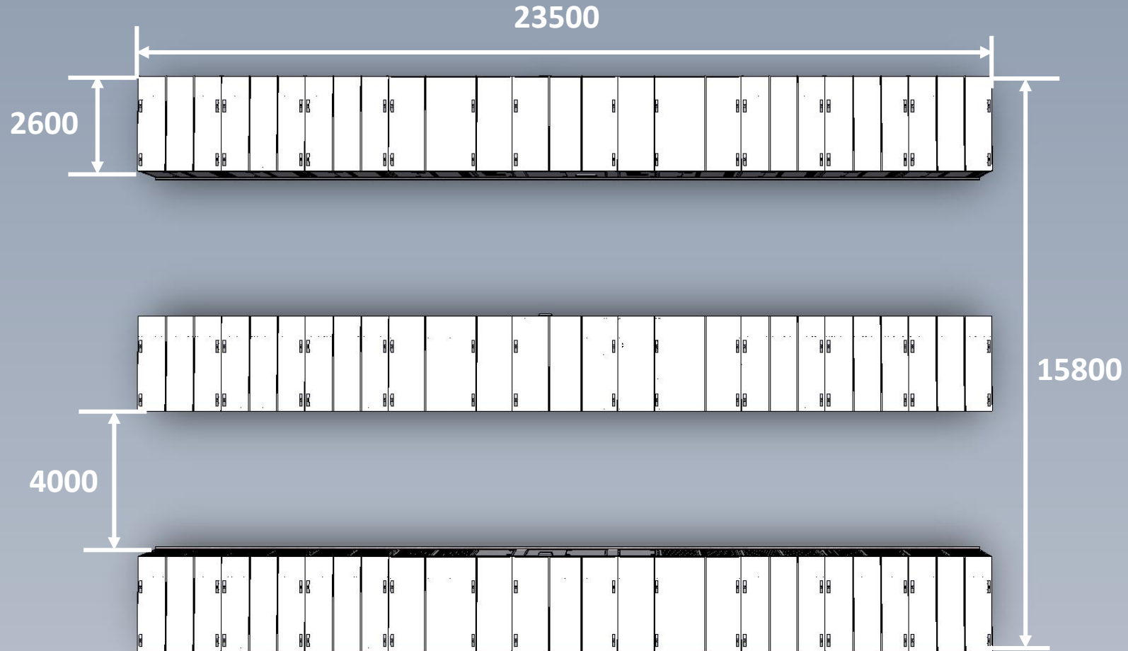
10MW/20MWh EMODULE P2 Hybrid energiavarastojärjestelmän layout ja alustavat mitat
